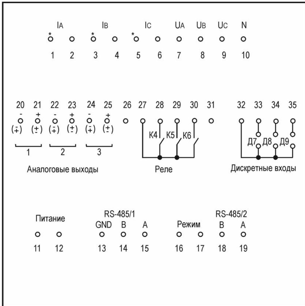
Рисунок В.1 - Схема подключения приборов
